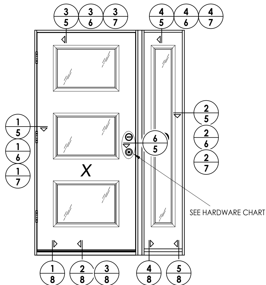
ELEVATION XO
