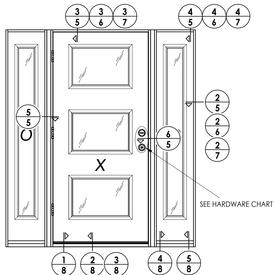
ELEVATION OXO
